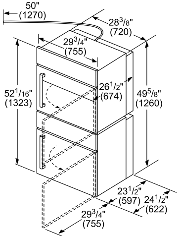
30" SideOpening Right Swing Door
