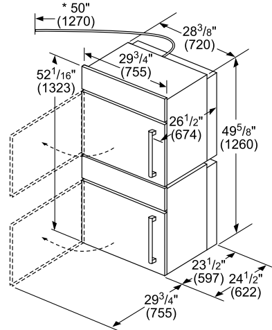
30" SideOpening Left Swing Door
