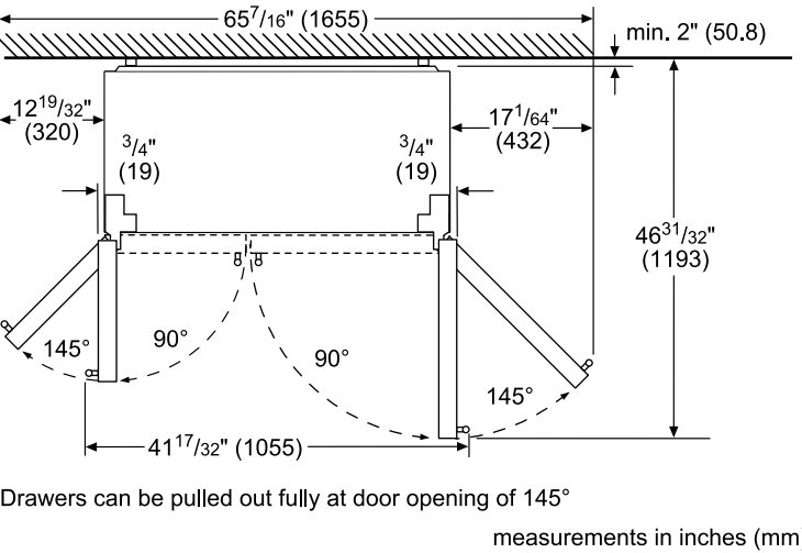
B20CS30SNS Dimensions (Overhead Views)
