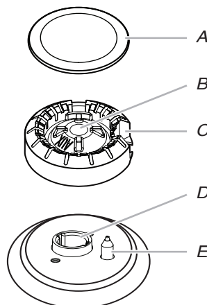
A. Chapeau de brûleur B. Ouverture du tube d'arrivée de gaz C. Base du brûleur D. Support d'injecteur E. Électrode d'allumage
