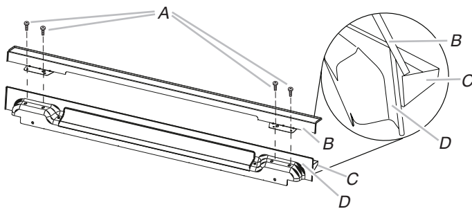
A. Vis n° 8-18 x 1/4" B. Déflecteur pour tiroir-réchaud C. Évent
