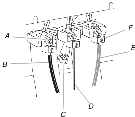
A. Écrou hexagonal 10-32 B. Ligne 2 (rouge) C. Vis de liaison à la terre D. Conducteur de mise à la terre nu (vert) E. Ligne 1 (noir) F. Cousse
