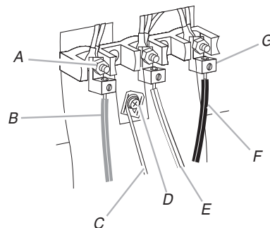
A. Tuerca hexagonal 10-32 B. Línea 2 (roja) C. Hilo desnudo de conexión a tierra (verde) D. Tornillo de puesta a tierra E. Hilo neutro (blanco) F. Línea 1 (negra) G. Lengüeta de terminal
